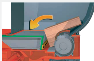
ホッパ 大きな梁材等によるラムのブロックを回避
