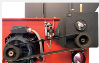
Vロータ駆動部 モータ22kW以下
